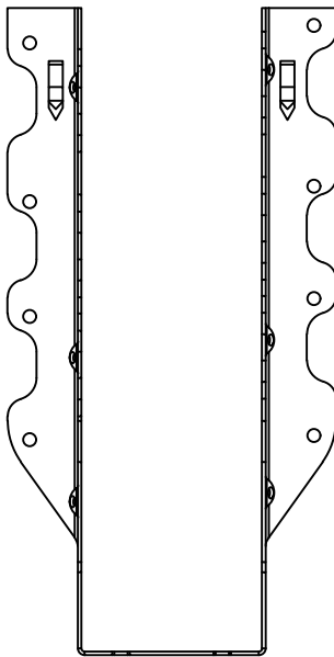
JUS310 - FRONT VIEW
